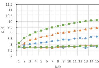
図2 ポンド模擬槽pH変化(流入pH11)
