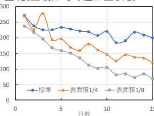
図4 ポンド模擬槽pH変化(流入pH11)
