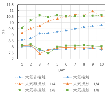
図4 ポンド模擬槽pH変化(流入pH11)
